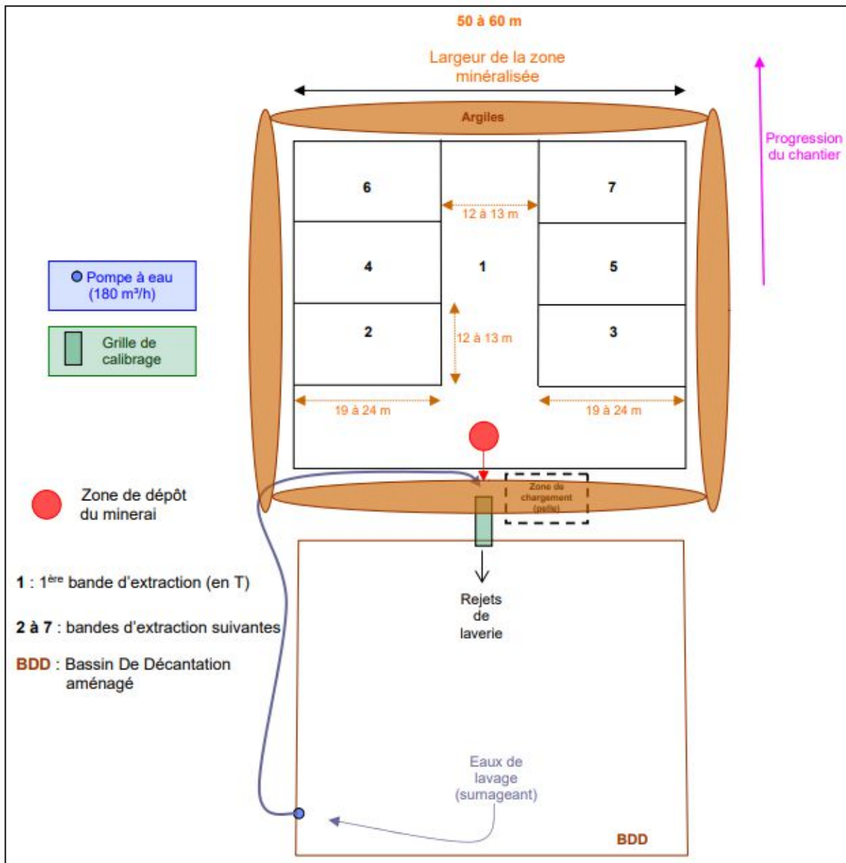
Figure 3 : Schéma de principe de l'exploitation envisagée par la SAS TERRE AVENIR
